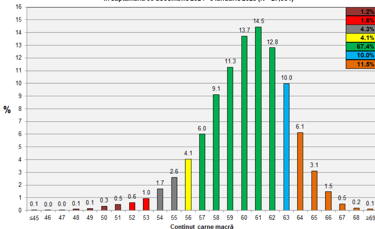
Distribuția conținutului de carne macră a carcaselor clasificate în România în săptămâna 30 decembrie 2024 - 5 ianuarie 2025 (N = 27,564)
