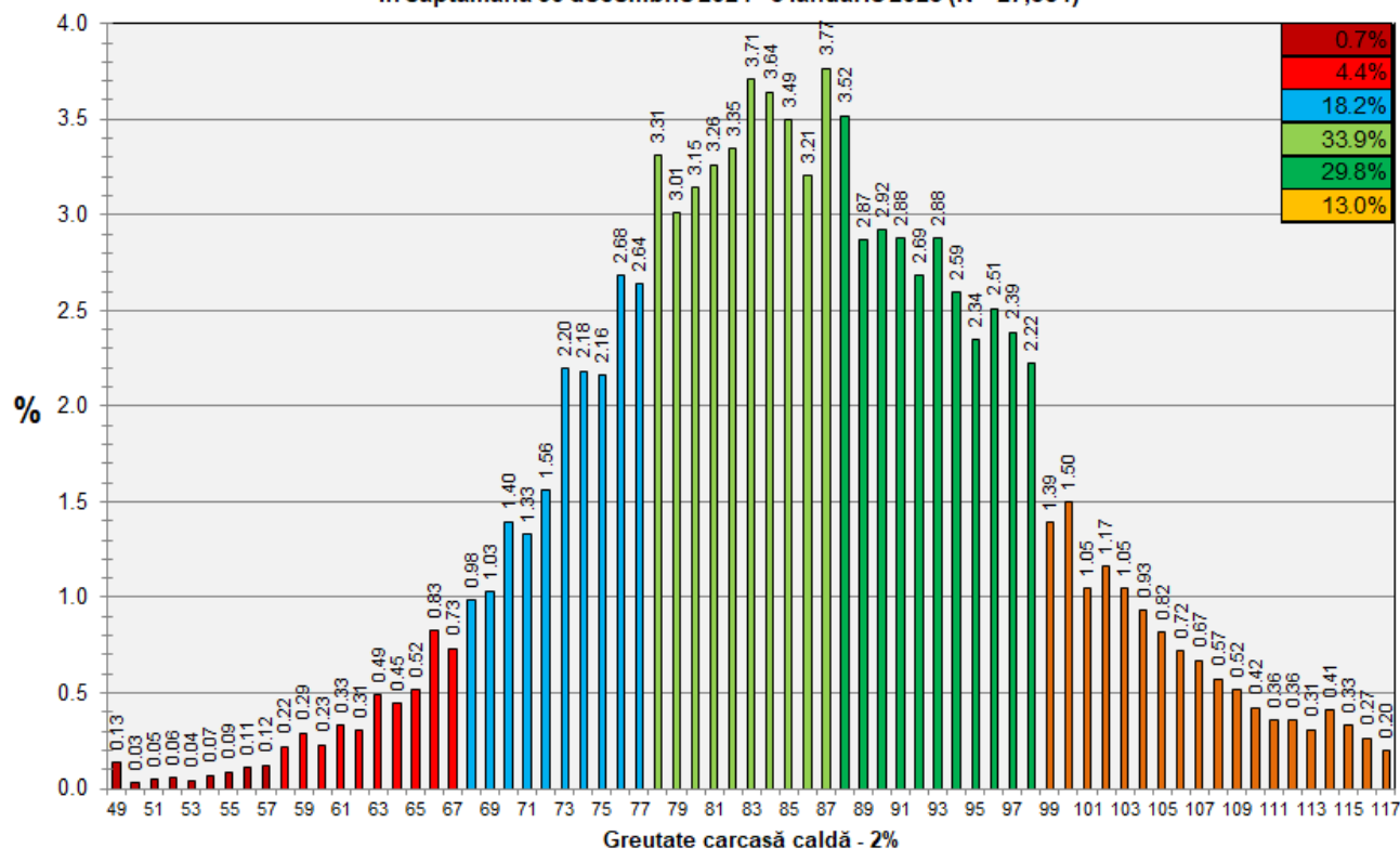
Distribuția greutatei carcaselor clasificate în România în săptămâna 30 decembrie 2024 - 5 ianuarie 2025 (N = 27,564)
