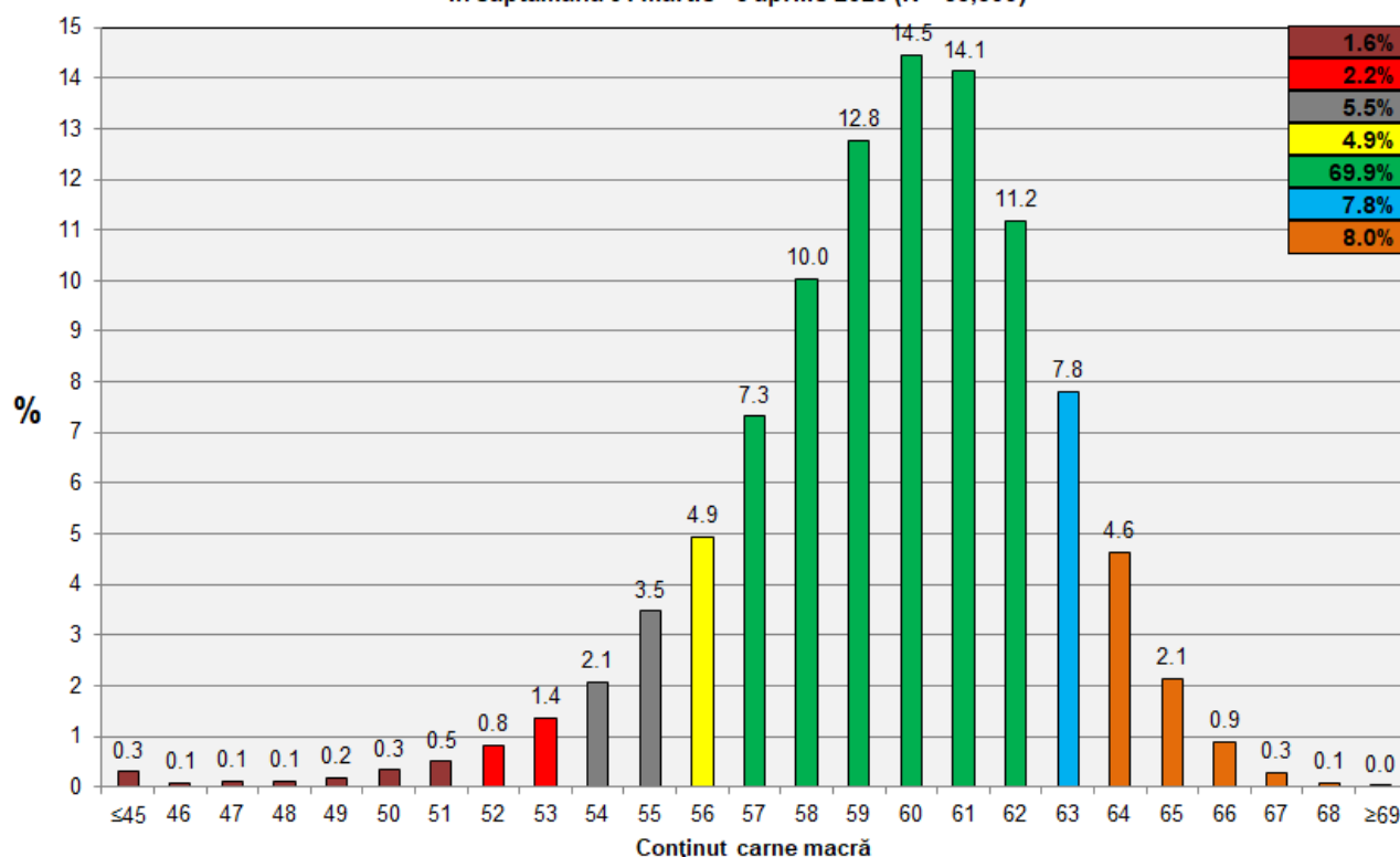
Distribuția conținutului de carne macră a carcaselor clasificate în România în săptămâna 31 martie - 6 aprilie 2025 (N = 65,599)
