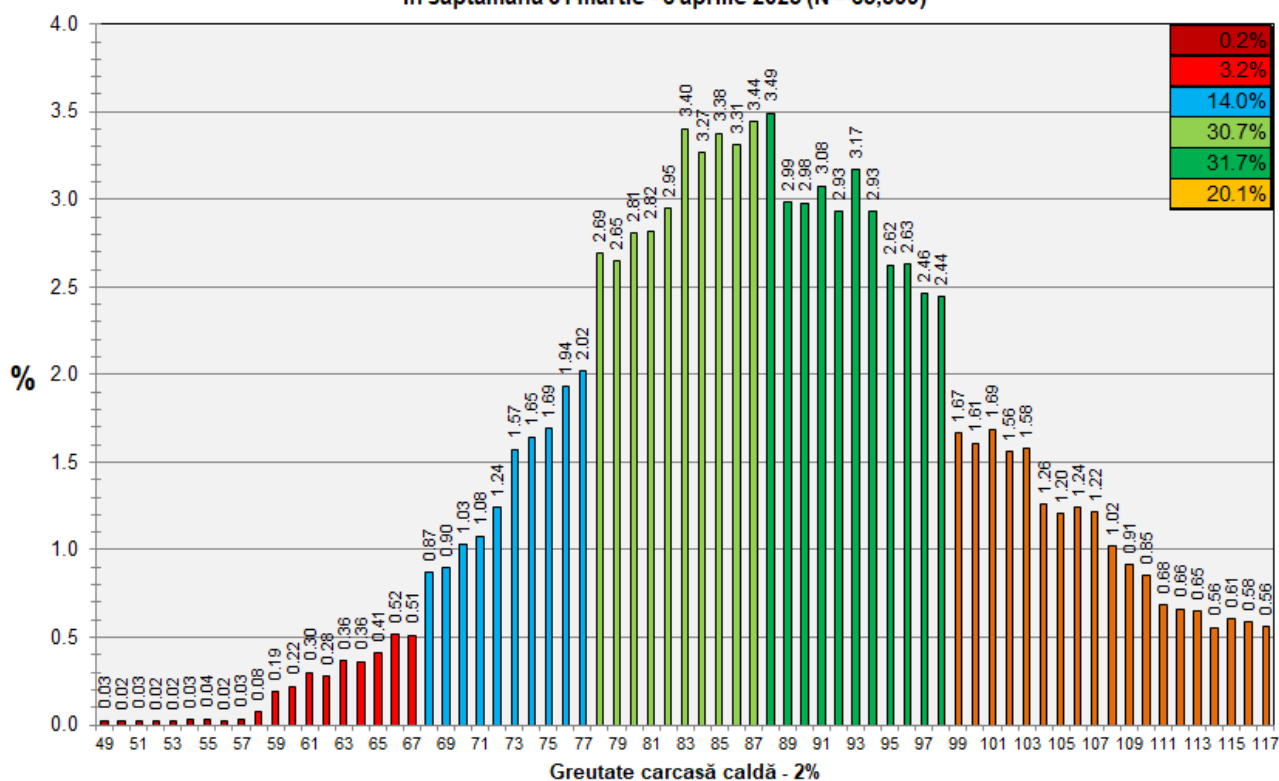
Distribuția greutatei carcaselor clasificate în România în săptămâna 31 martie - 6 aprilie 2025 (N = 65,599)
