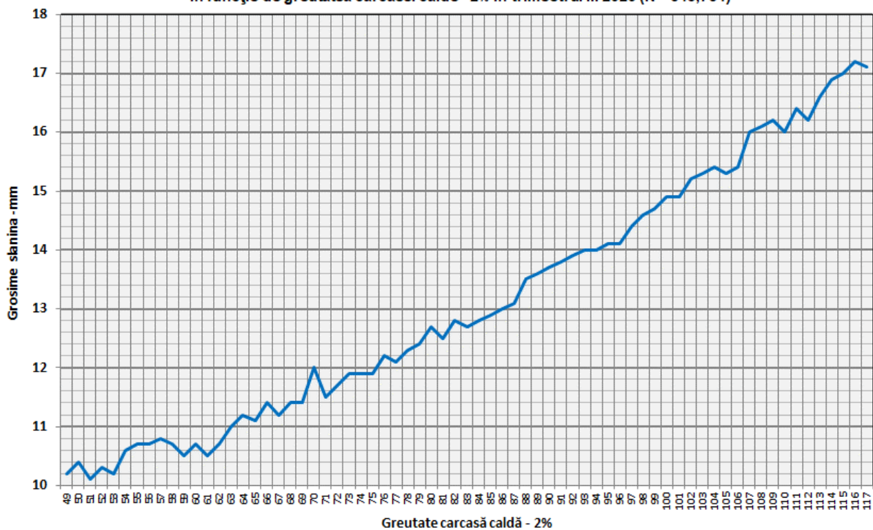
Grosimea slaninii cu echipamentul cu sondă optică OptiGrade-Pro în România în funcție de greutatea carcasei calde - 2% în trimestrul III 2023 (N = 645,764)
