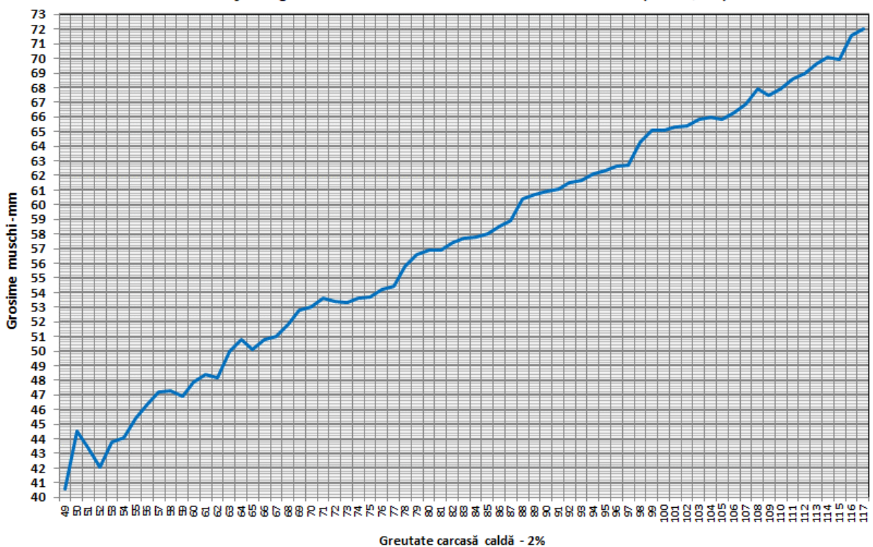
Grosimea muschiului cu echipamentul cu sondă optică Fat-O-Meater în România în funcție de greutatea carcasei calde - 2% în trimestrul III 2023 (N = 93,476)
