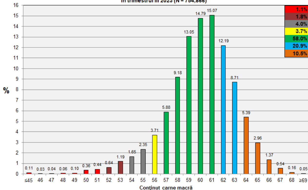
Distribuția conținutului de carne macră a carcaselor clasificate în România în trimestrul III 2023 (N = 754,866)
