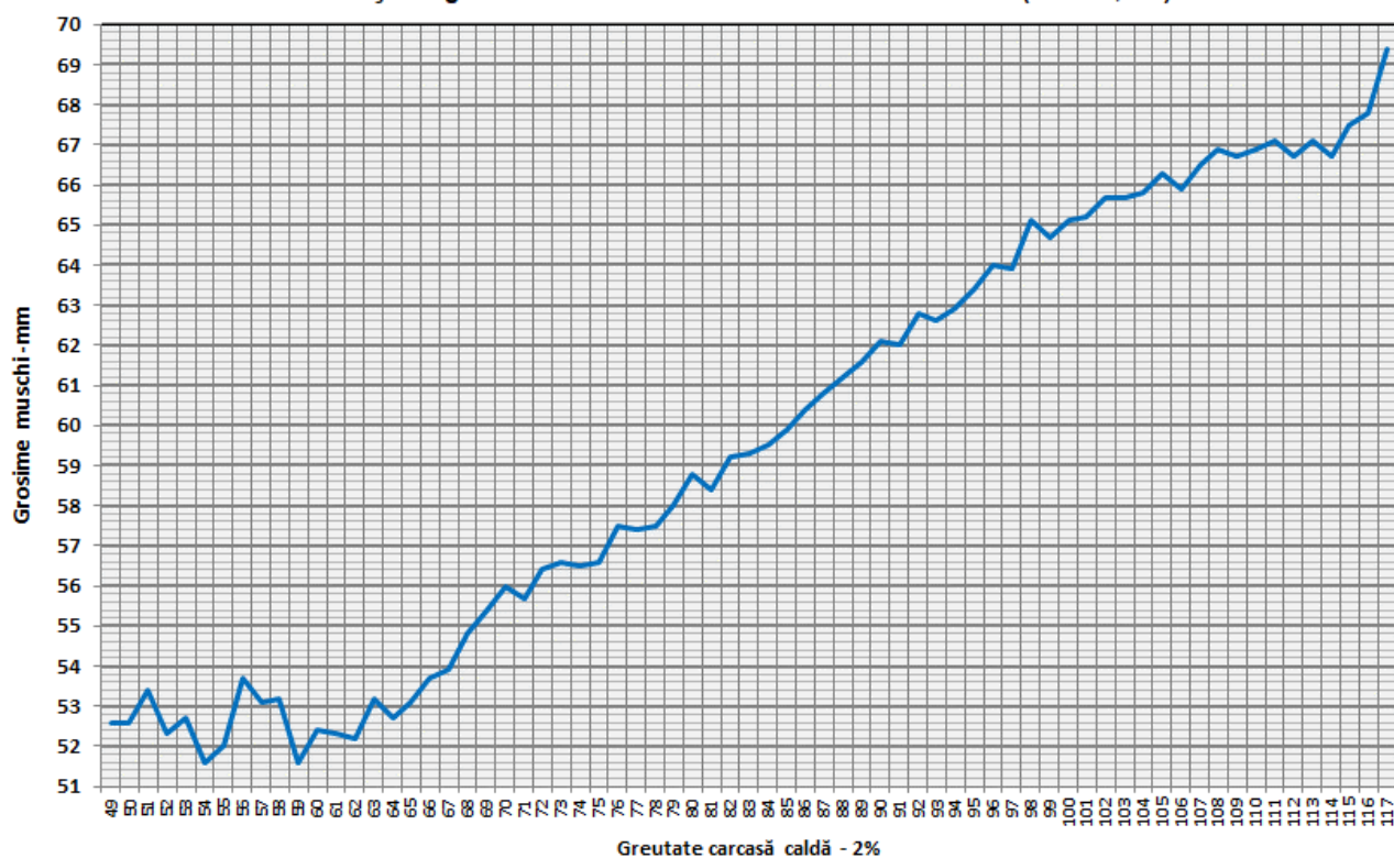
Grosimea muschiului cu echipamentul cu sondă optică OptiGrade-Pro în România în funcție de greutatea carcasei calde - 2% în trimestrul III 2023 (N = 645,764)
