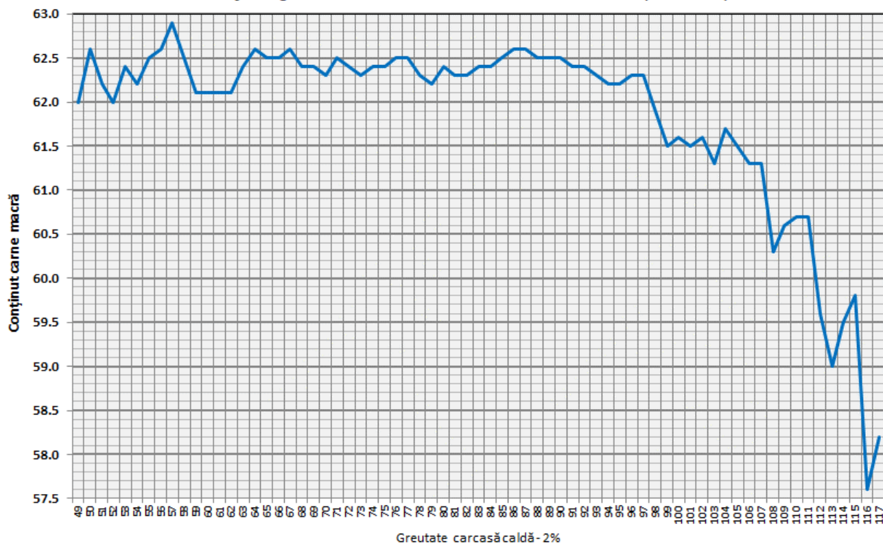
Conținutul de carne macră cu echipamentul cu sondă optică Fat-O-Meater în România în funcție de greutatea carcasei calde - 2% în trimestrul III 2023 (N = 93,476)
