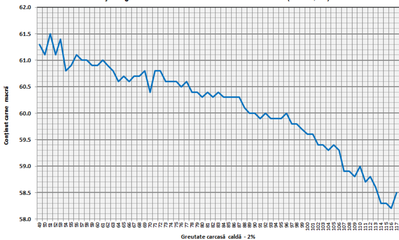
Conținutul de carne macră cu echipamentul cu sondă optică OptiGrade-Pro în România în funcție de greutatea carcasei calde - 2% în trimestrul III 2023 (N = 645,764)
