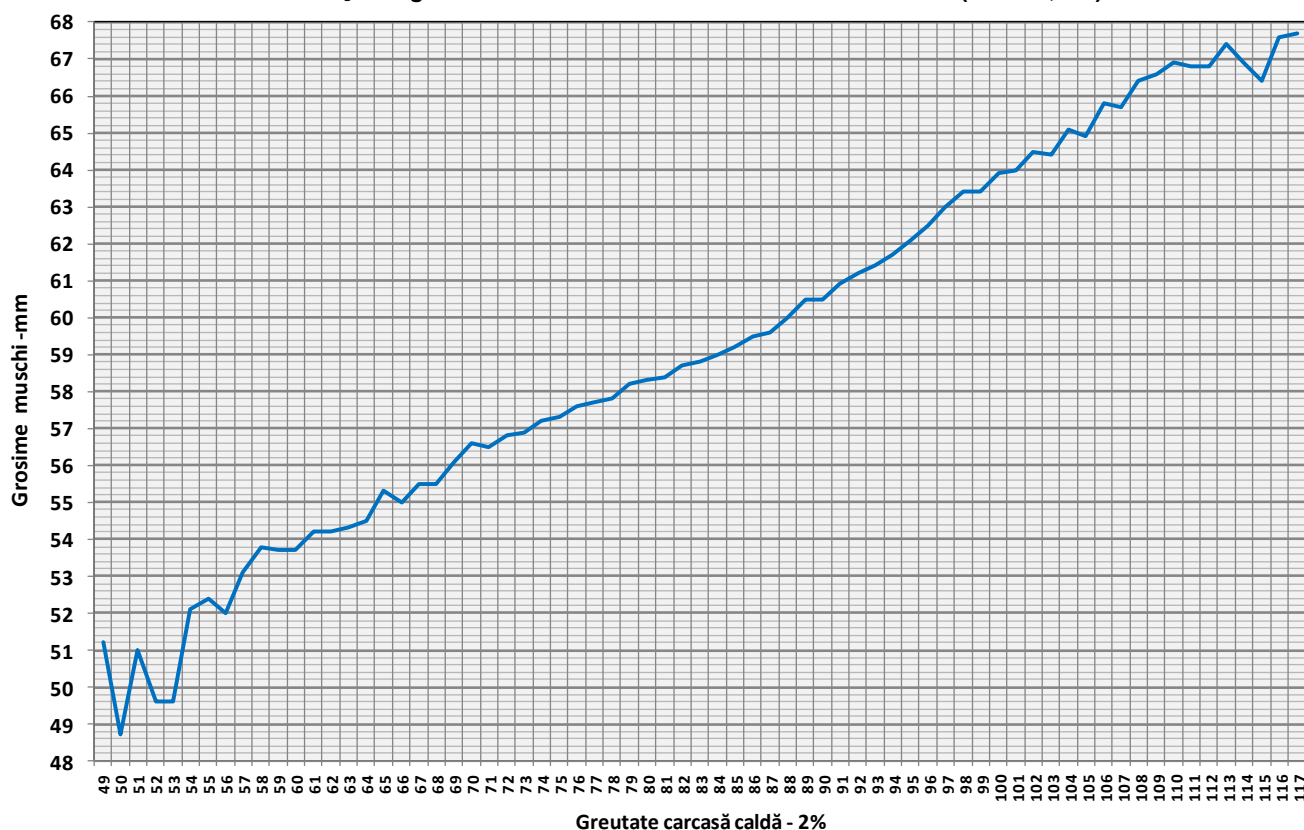
Grosimea muschiului cu echipamentul cu sondă optică OptiGrade-Pro în România în funcție de greutatea carcasei calde - 2% în trimestrul III 2019 (N = 797,835)
