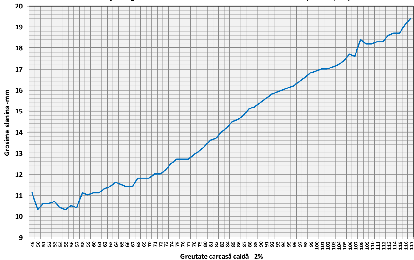
Grosimea slaninii cu echipamentul cu sondă optică OptiGrade-Pro în România în funcție de greutatea carcasei calde - 2% în trimestrul III 2018 (N = 790,582)
