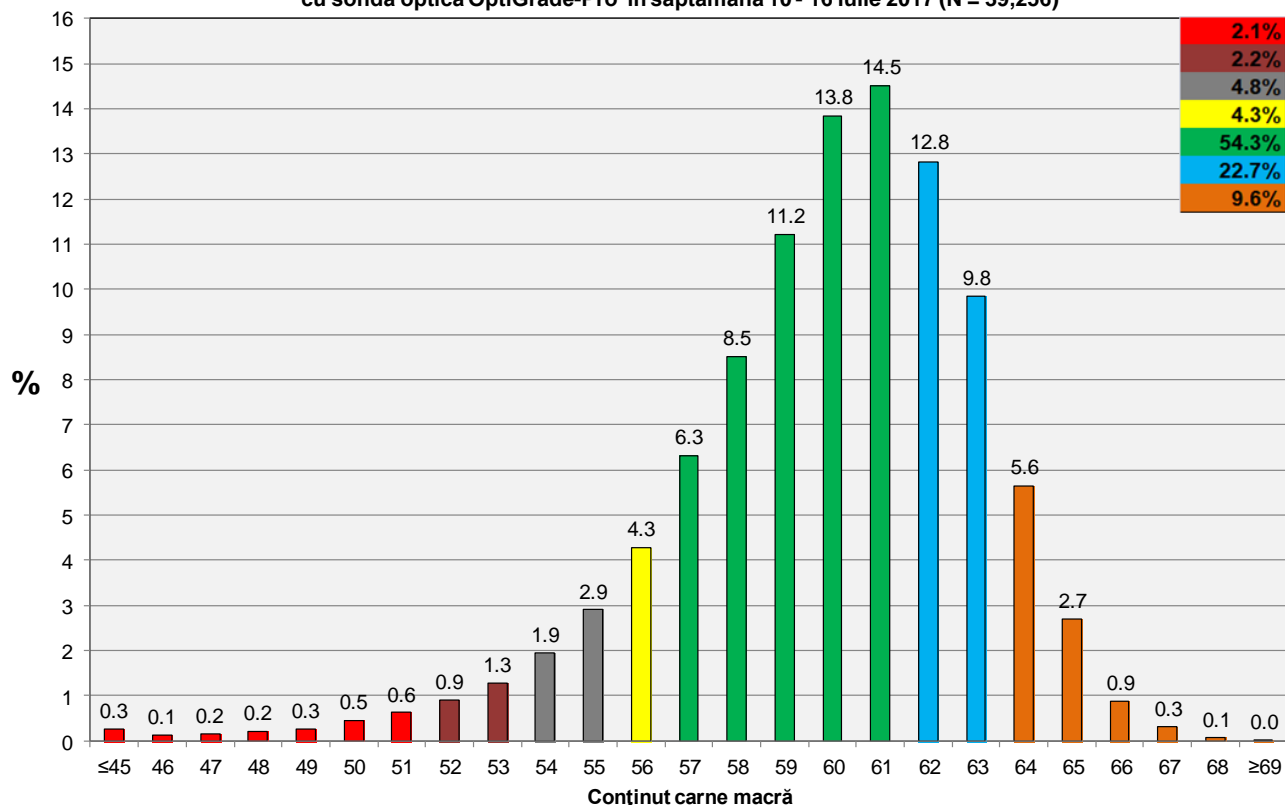
Distribuția conținutului de carne macră a carcaselor clasificate în România cu echipamentul cu sondă optică OptiGrade-Pro în săptămâna 10 - 16 iulie 2017 (N = 39,256)
