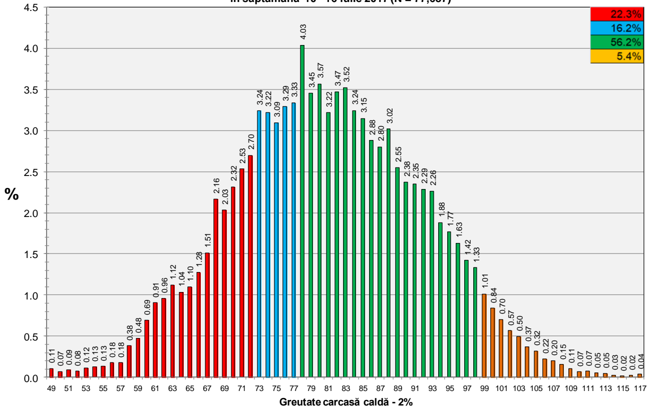
Distribuția greutății carcaselor clasificate în România în săptămâna 10 - 16 iulie 2017 (N = 77,687)
