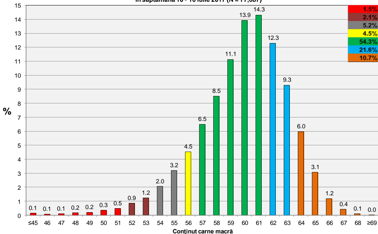
Distribuția conținutului de carne macră a carcaselor clasificate în România în săptămâna 10 - 16 iulie 2017 (N = 77,687)
