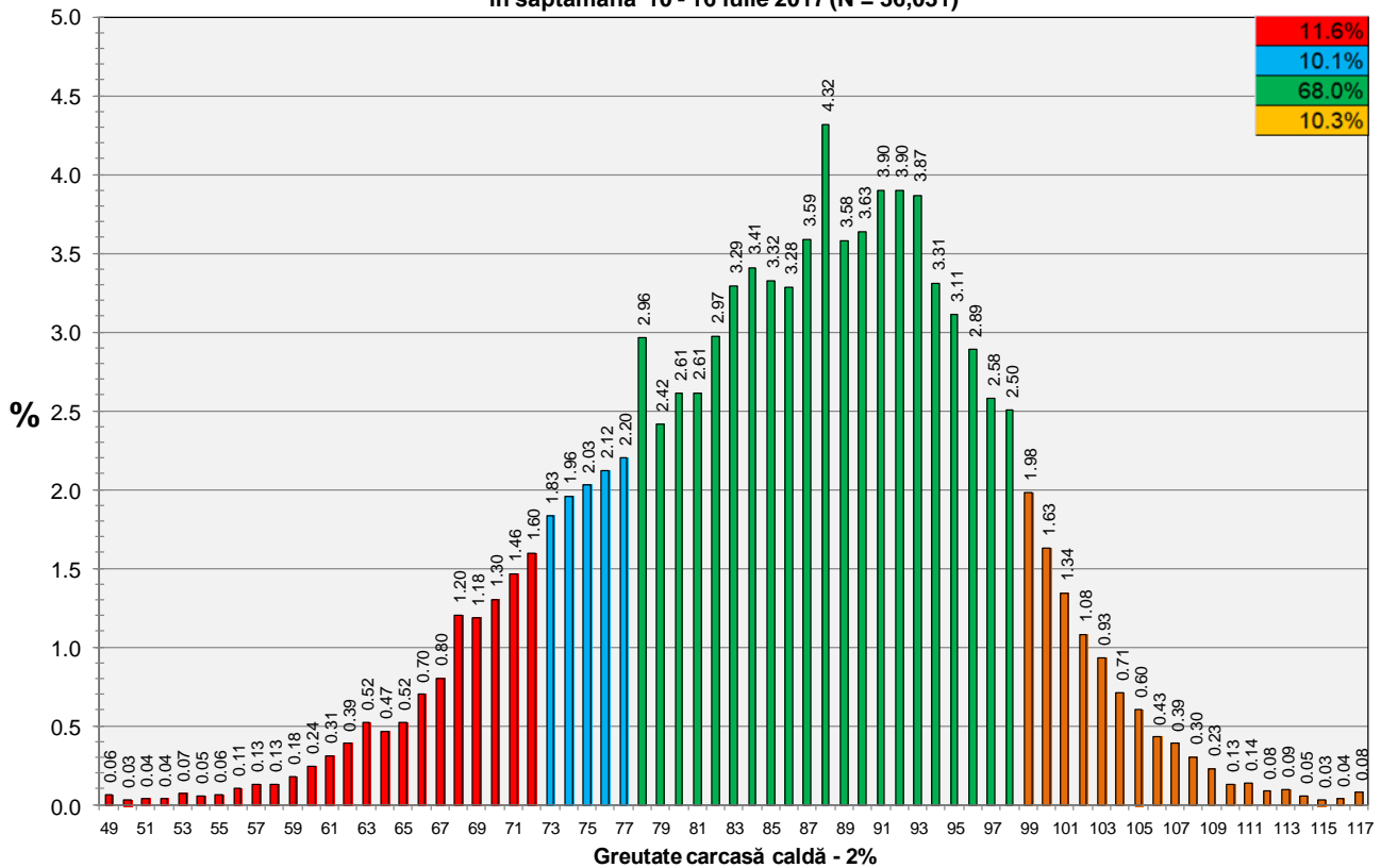
Distribuția greutății carcaselor clasificate în România cu echipamentul cu sondă optică Fat-O-Meater în săptămâna 10 - 16 iulie 2017 (N = 36,031)
