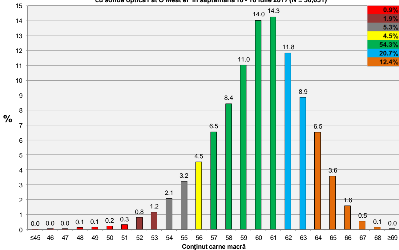
Distribuția conținutului de carne macră a carcaselor clasificate în România cu echipamentul cu sondă optică Fat O Meat'er în săptămâna 10 - 16 iulie 2017 (N = 36,031)
