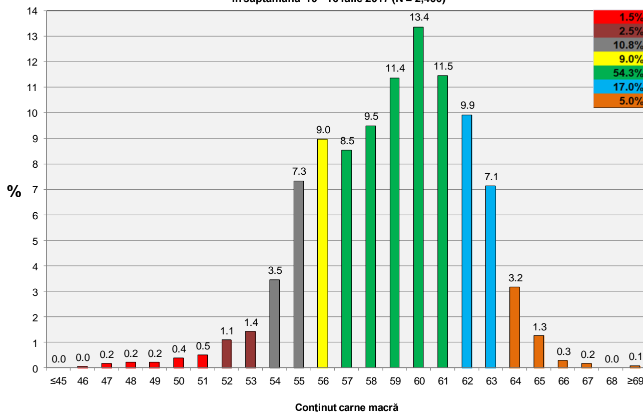
Distribuția conținutului de carne macră a carcaselor clasificate în România cu metoda ZP în săptămâna 10 - 16 iulie 2017 (N = 2,400)
